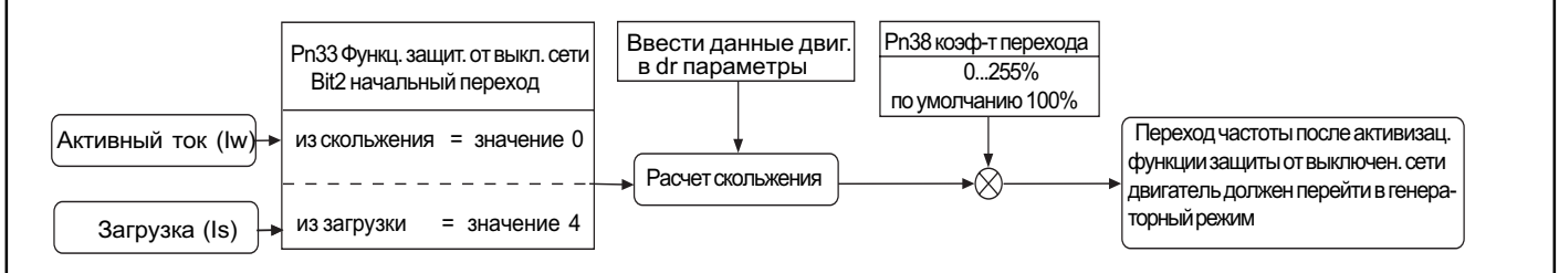
Рис. 6.9.3.б Переход частоты для генераторного режима
