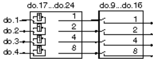
Рис. 6.3.16 Инвертирование и выбор условий коммутации
