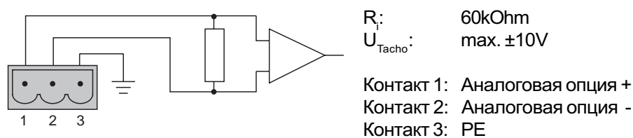
Рис. 6.10.4.b Схема подключения для входа ±10V
