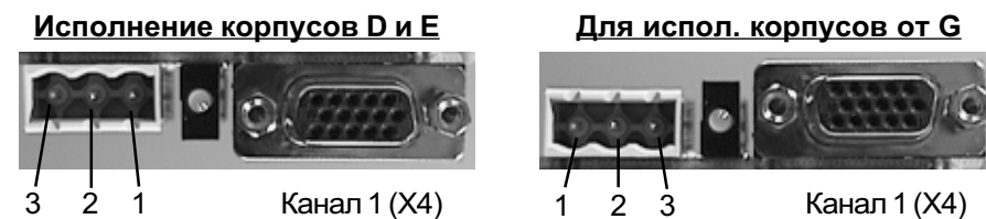
Рис. 6.10.4.a Интерфейс дискретного датчика с инициатором входа
