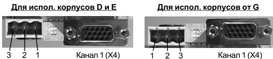
Рис. 6.10.3.a Интерфейс датчика перемещения с тахогенератором
