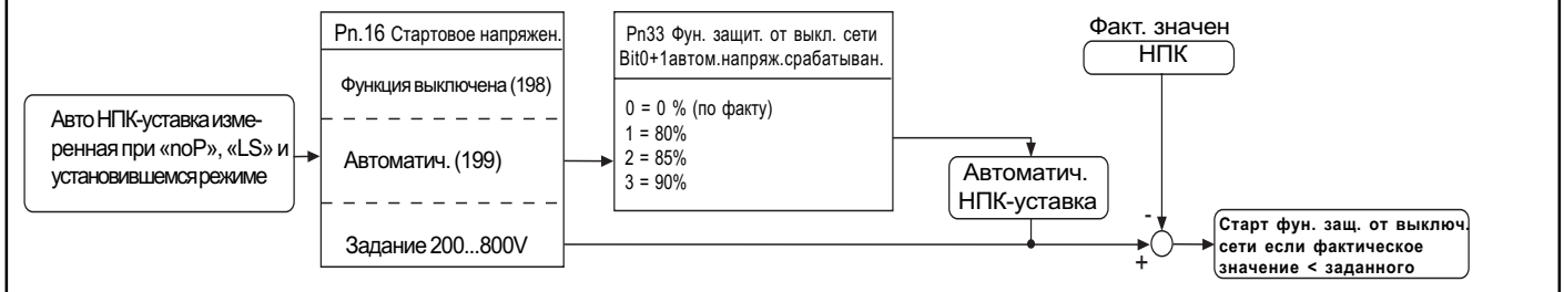
Рис. 6.9.3.а Включение функции защиты от выключения сети (ЗВС)
