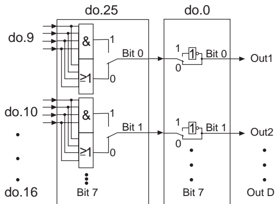
Рис. 6.3.18 Объединение условий коммутации и инвертирование выходов
