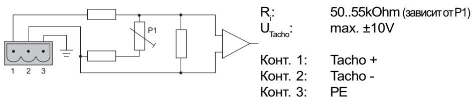
Рисонок 6.10.3.b Схема подключения тахогенератора
