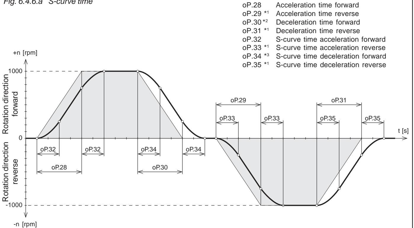
Fig. 6.4.6.a S-curve time
