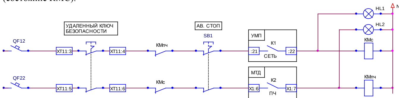
Рисунок 2.2.2. Цепи управления контакторами.
