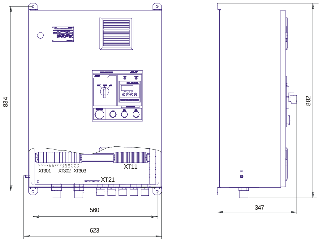
Габаритно-присоединительный чертеж типоразмеры СМП122-011х1...СМП122-022х1.
