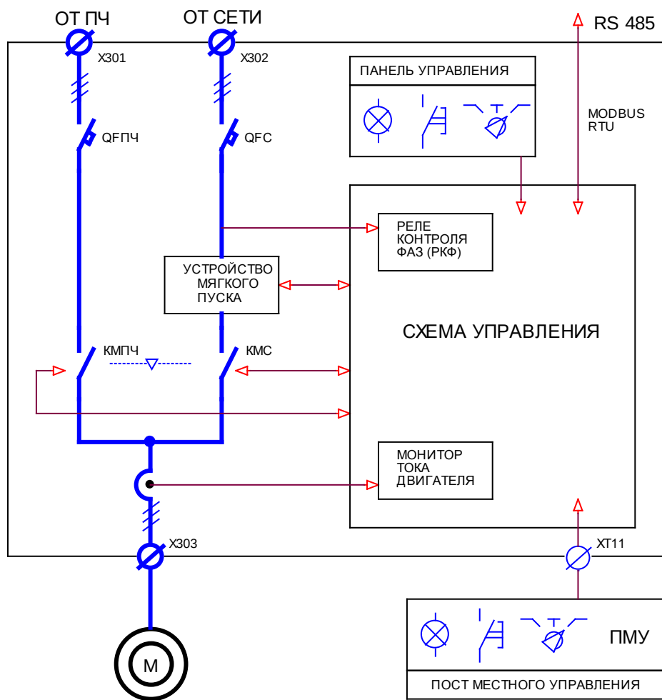
Рисунок 1.1.1. Функциональная схема СМП122.
