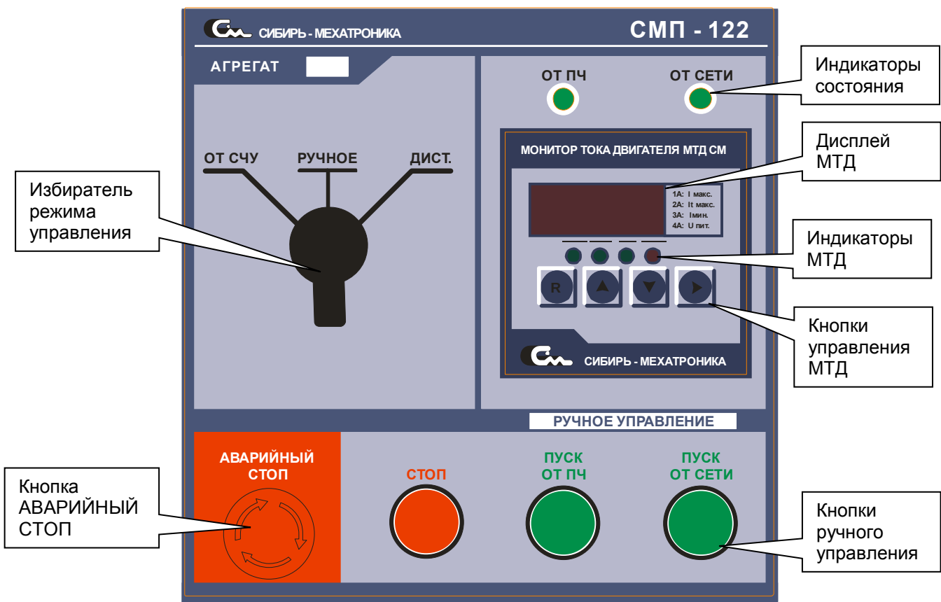
Рисунок 2.4.1. Панель управления. Внешний вид.
