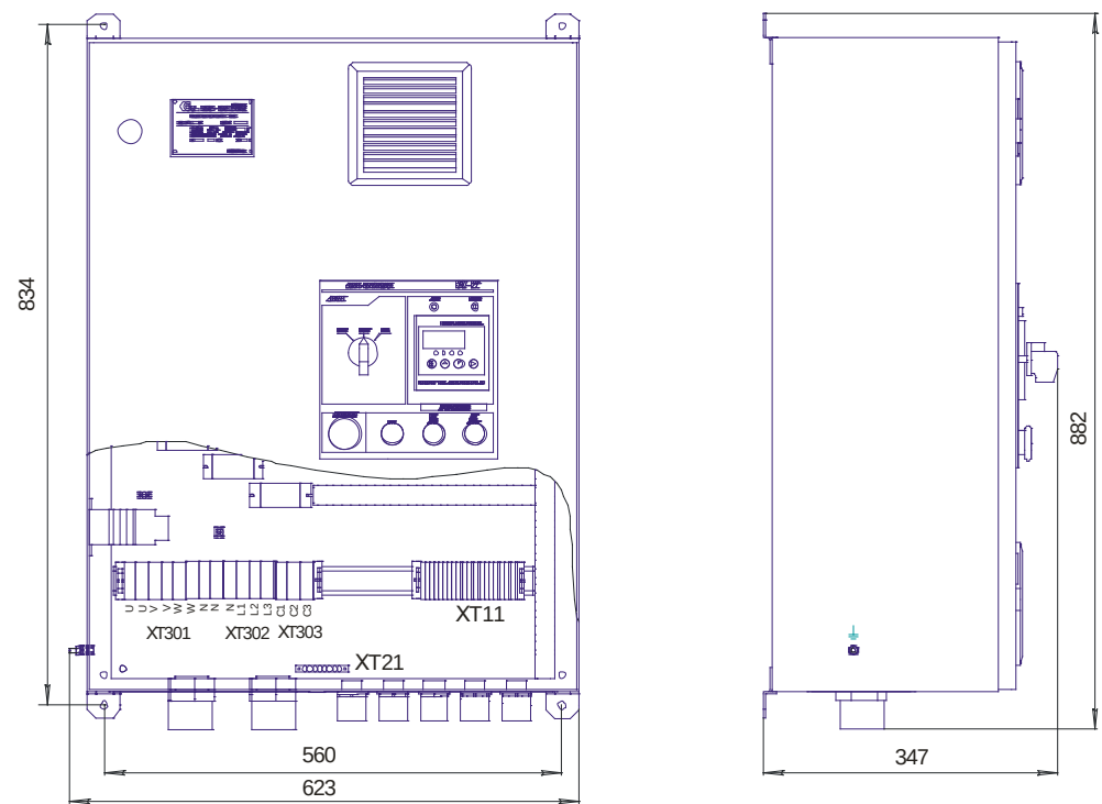
Габаритно-присоединительный чертеж типоразмеры СМП122-030х1...СМП122-037х1.
