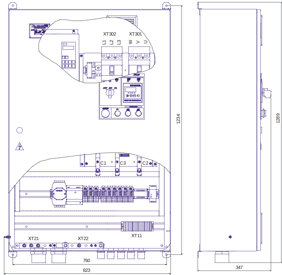
Габаритно-присоединительный чертеж типоразмеры СМП122-075х1...СМП122-090х1.
