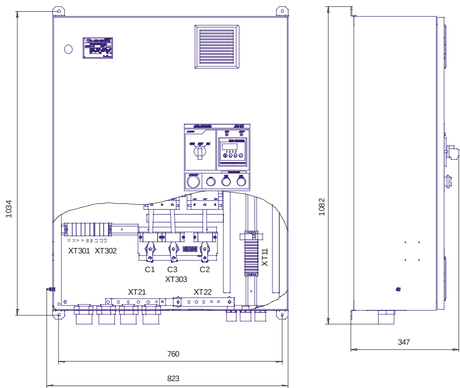
Габаритно-присоединительный чертеж типоразмеры СМП122-045х1...СМП122-055х1.
