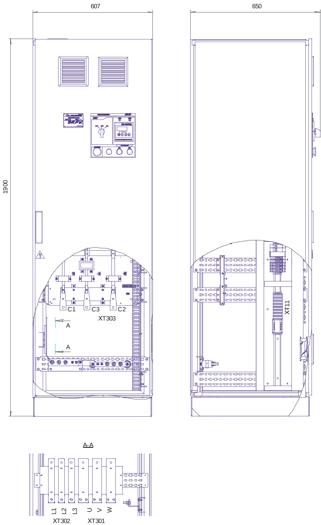
Габаритно-присоединительный чертеж типоразмеры СМП122-110х1...СМП122-132х1.
