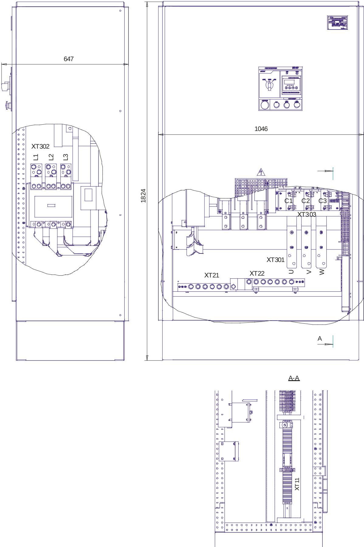
Габаритно-присоединительный чертеж типоразмеры СМП122-250х1...СМП122-315х1.
